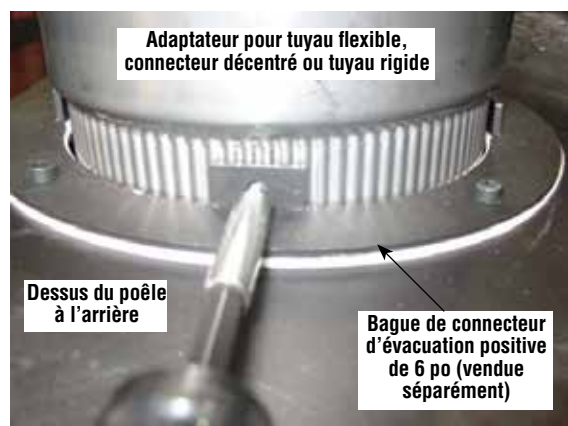
Figure 7 - Bague de connecteur
