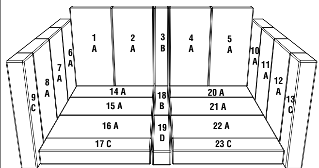
Disposition des briques de la boîte à feu vue depuis l'avant
