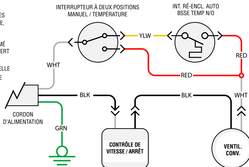
Figure 36 - ML230GL Schéma de câblage du ventilateur
