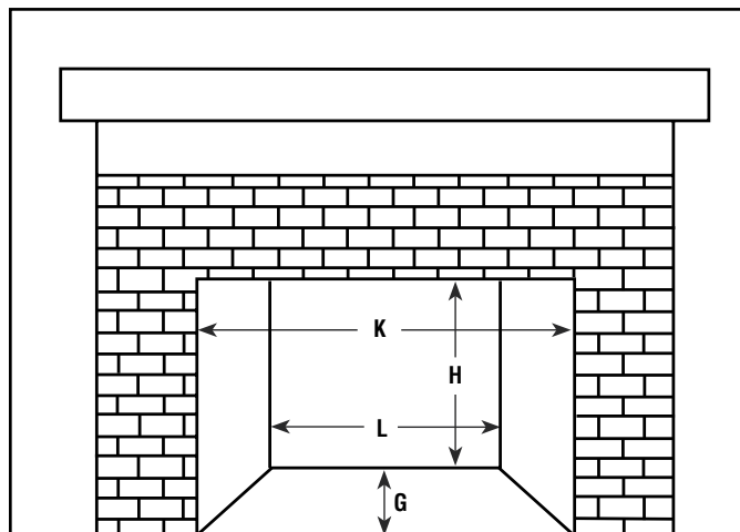
Figure 4 - Cavité minimum pour le foyer
