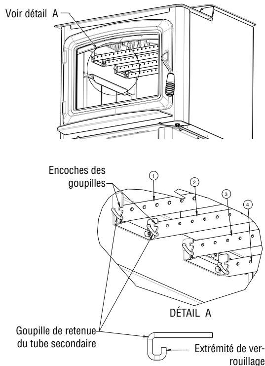
Figure 26 - Dispositifs de fixation des tubes d'air secondaires
