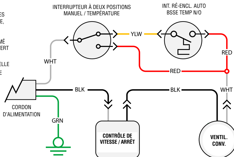
Figure 28 - ML300 Schéma de câblage du ventilateur
