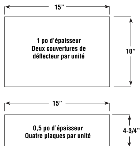
Figure 3 - Pièces d'isolation du déflecteur
