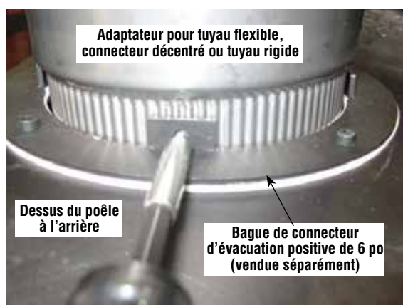
Figure 8 - Bague de connecteur
