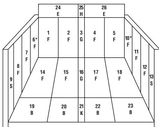
Disposition des briques de la boîte à feu vue depuis l'avant
