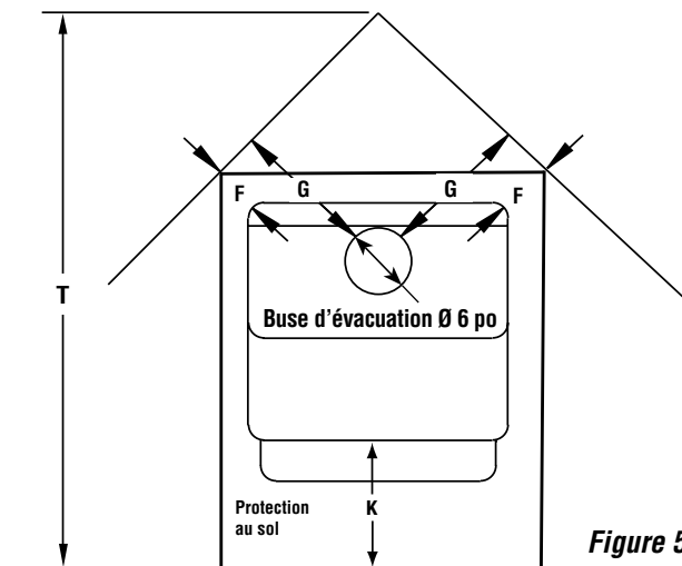
Figure 4 : Dégagement de coin, poêle et conduit au mur – Vue de dessus
